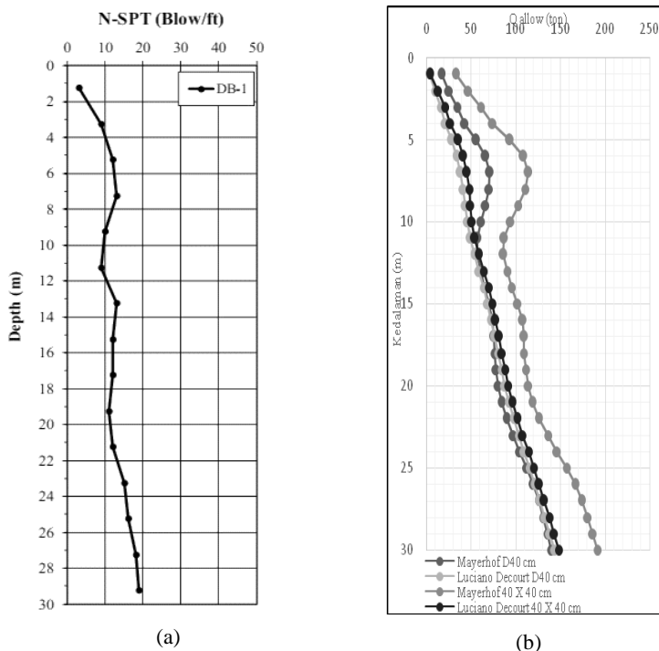
Gambar 1. a) Data NSPT b)Grafik hubungan Q allow dengan kedalaman
