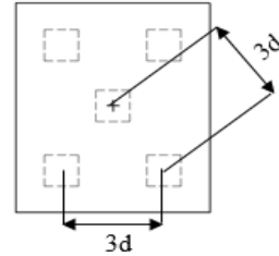
Gambar 2. Konfigurasi 5 tiang
