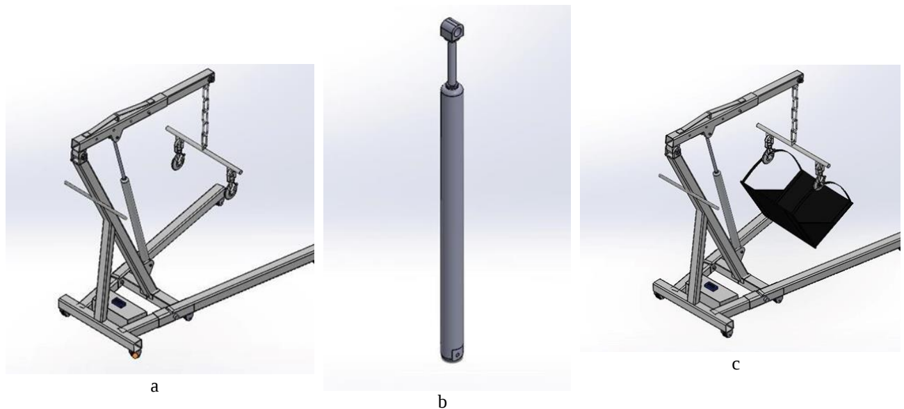
Gambar 2. a) Desain Linier Actuator b) Desain Rangka c) Crane saat digunakan
