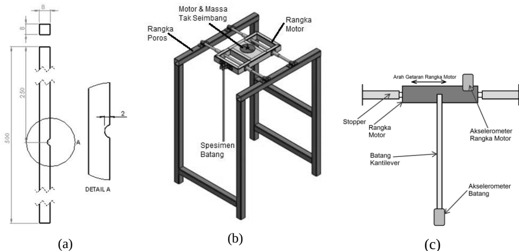
Gambar 1. a) Spesimen batang, b) mesin penggetar, c) penempatan akselerometer.
