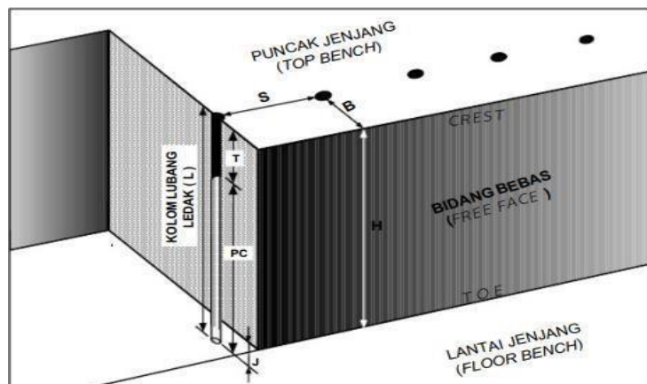
Gambar 2. Geometri Peledakan C.J.Konya
