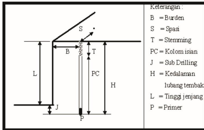
Gambar 1. Geometri Peledakan R.L.Ash
