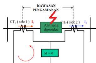
Gambar 2. Kondisi Gangguan Dalam Differential Relay [1]
