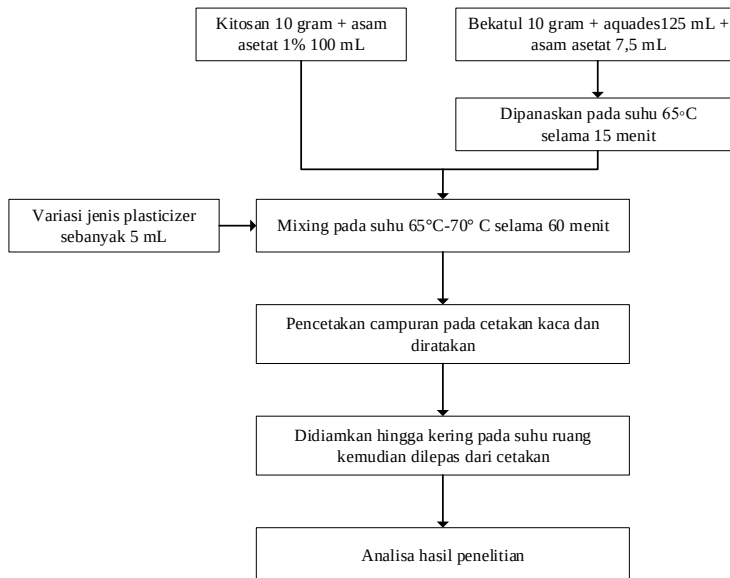
Gambar 1. Alur Pembuatan Plastik Biodegradable
