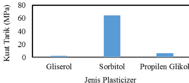
Gambar 3. Grafik Hasil Uji Kuat Tarik dengan Variasi Jenis Plasticizer
