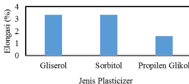
Gambar 3. Grafik Hasil Uji Elongasi dengan Variasi Jenis Plasticizer
