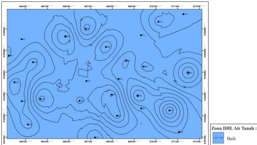
Gambar 4. Peta nilai Daya Hantar Listrik (DHL) di lokasi penelitian
