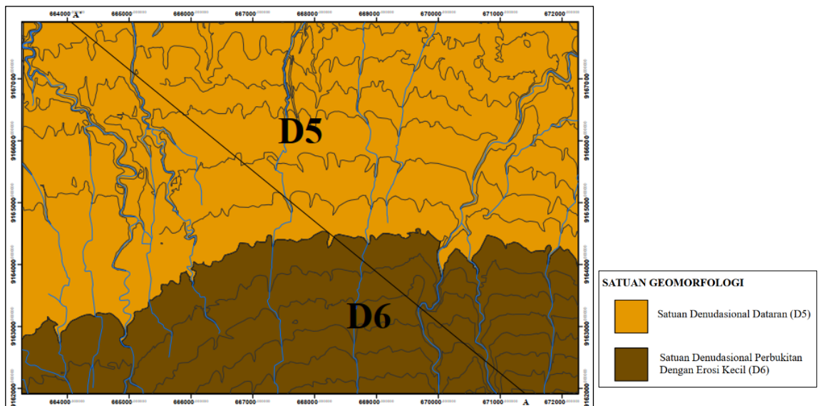
Gambar 2. Peta Satuan Geomorfologi lokasi penelitian
