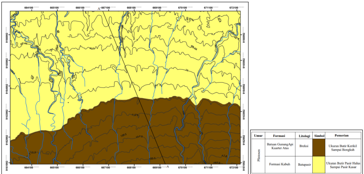
Gambar 3. Peta Satuan Geologi lokasi penelitian
