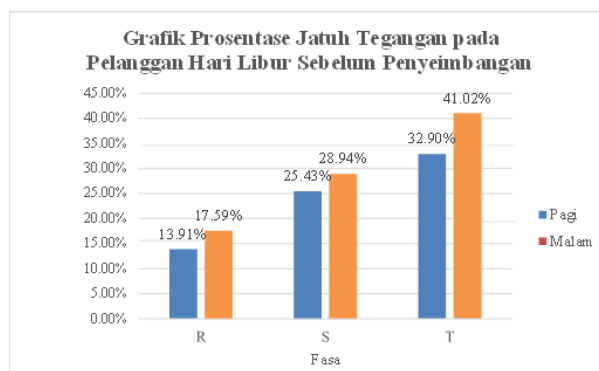
Gambar 5. Grafik Prosentase Jatuh Tegangan Antar Fasa sebelum Penyeimbangan
