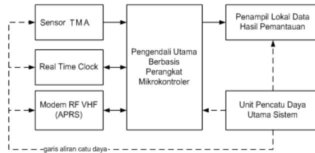
Gambar 2. Blok Diagram Pemantau Tinggi Muka Air
