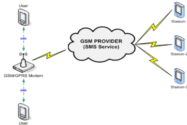
Gambar 3. Konfigurasi GSM Gateway
