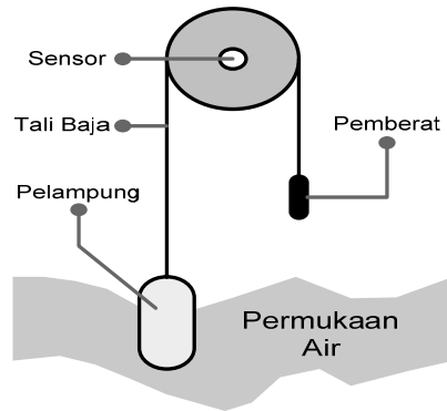
Gambar 1. Model Pengukuran Teknik Pelampung
