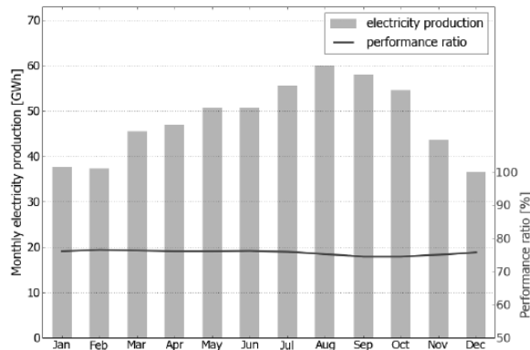
Gambar 3. Produksi energi listrik dan performance ration bulanan
