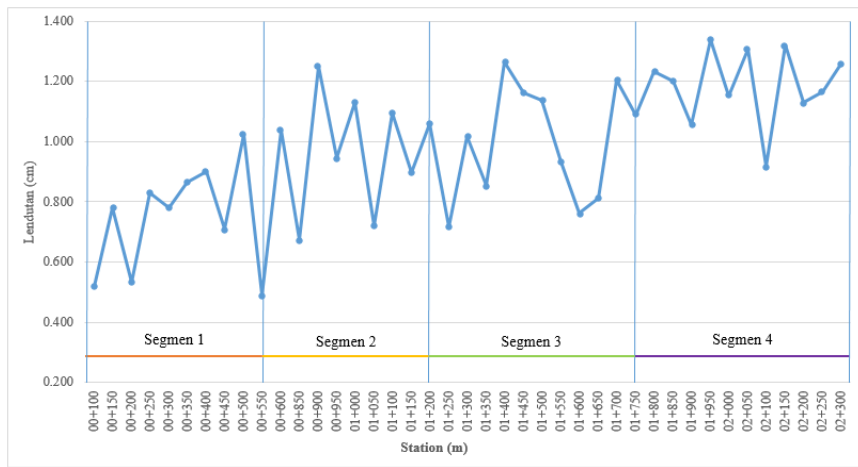
Gambar 3. Grafik Lendutan Balik
