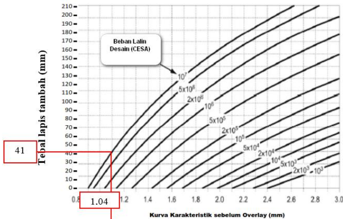
Gambar 4. Solusi Overlay Berdasarkan Lendutan Benkelman Beam Untuk WMAPT 41°C Menentukan Overlay dengan Curva Lendutan Untuk Mencegah Retak Fatigue
