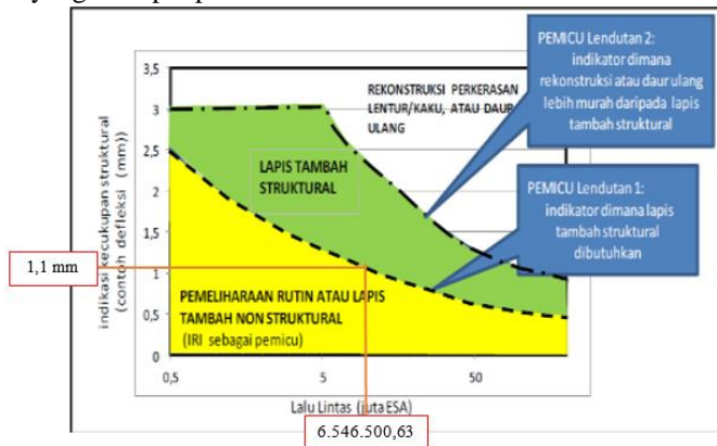
Gambar 2. Pemicu Konseptual Untuk Penanganan Perkerasan
