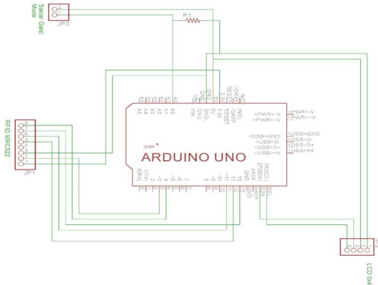
Gambar 2 Rancangan Kabel
