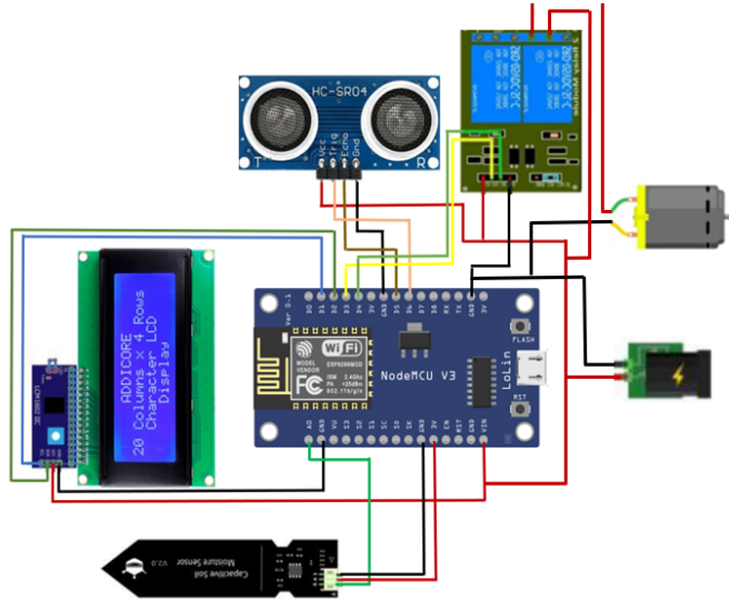
Gambar 2. Wiring Diagram Penyiraman Otomatis
