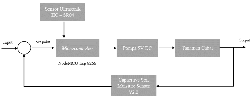
Gambar 1. Blok Diagram Sistem Penyiraman
