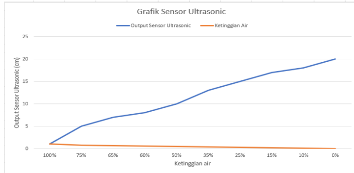
Gambar 6. Grafik Sensor Ultrasonic
