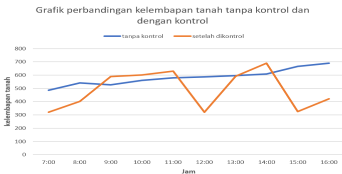
Gambar 7. Grafik perbandingan kelembapan tanah sebelum dikontrol dan setelah dikontrol
