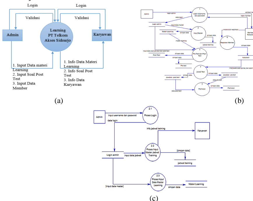
Gambar 1. a) Konteks Diagram, b) DFD Level 0, c) DFD Level 1
