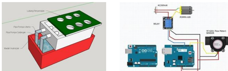
Gambar 1. Rancangan rangkaian sistem penanaman hidroponik dan Elektronika
