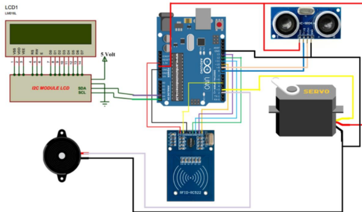
Gambar 1. Skematik Rangkaian Sistem
