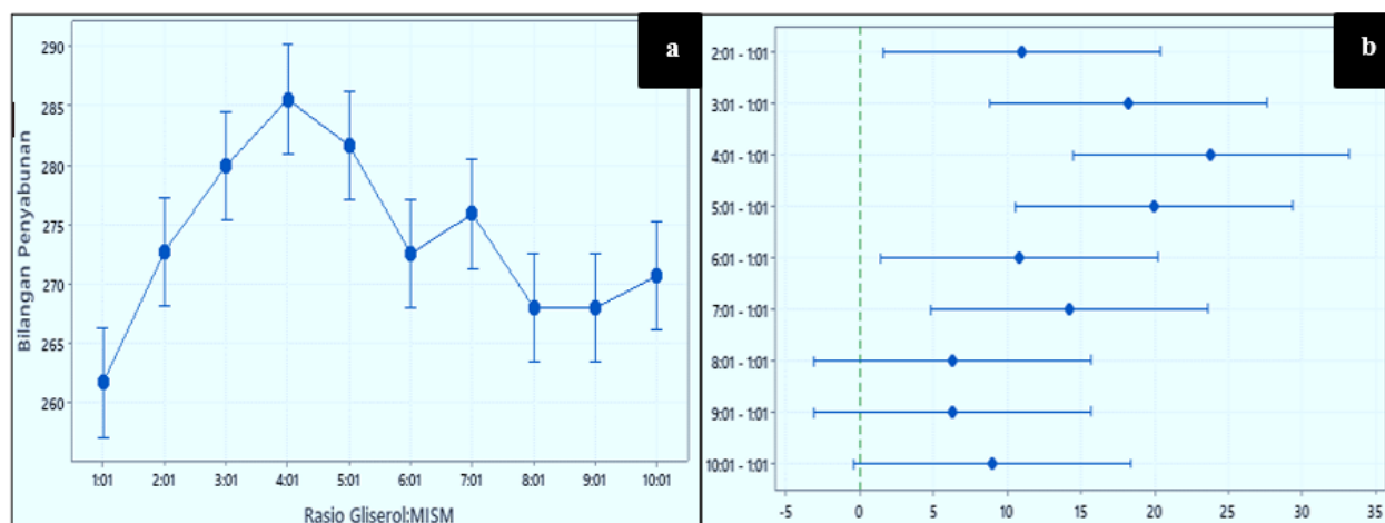
Gambar 5. Korelasi Konsentrasi Gliserol : MISM (Mol) Terhadap Bilangan Penyabunan MDAG
