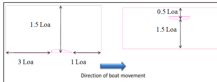
Gambar 7. Ukuran Panjang Domain
