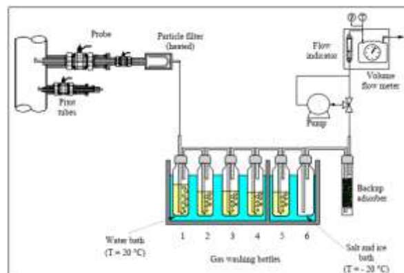
Gambar 3. Rangkaian pengambilan sampel tar
