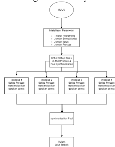
Gambar 4. Process parallel pada ACO dengan metode synchronization pool
