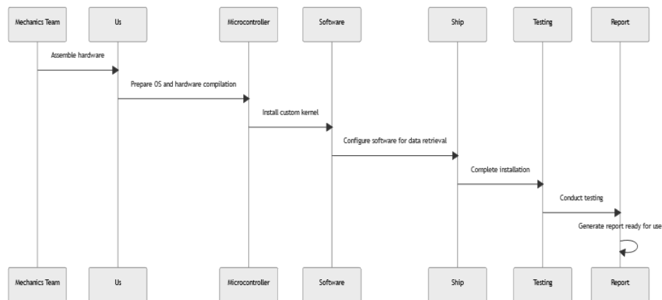
Gambar 1. Alur Pemasangan
