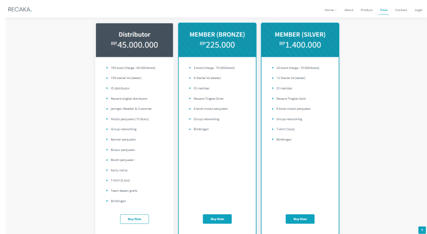
Gambar 6. Halaman Utama
