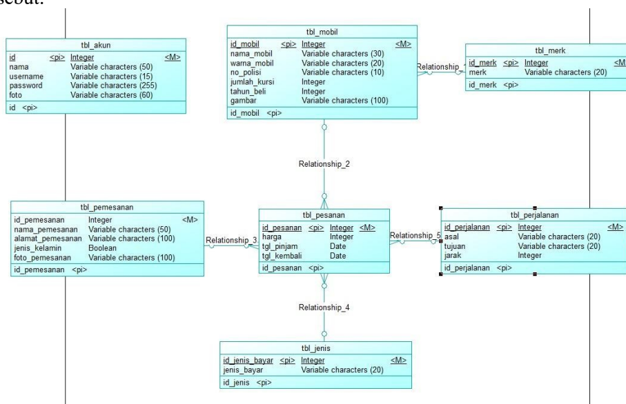
Gambar 4. Gambar Desain Database Cdm.
