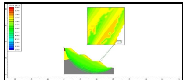
Gambar 2: Contoh Permodelan Lereng Keseluruhan, Tinggi = 8 meter, dan sudut = 40°
