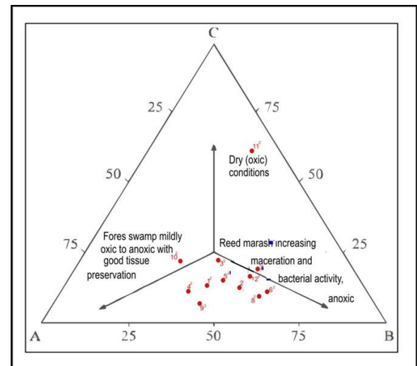
Gambar 6: Plotting maseral Seam-X terletak pada kondisi oxic-anoxic (Mukopadhyay et al., 1991)
