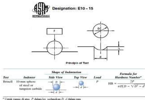
Gambar 3: Pengujian Kekerasan Brinell Standar ASTM E10
