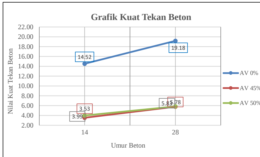
Gambar 4. Grafik Kuat Tekan Beton
