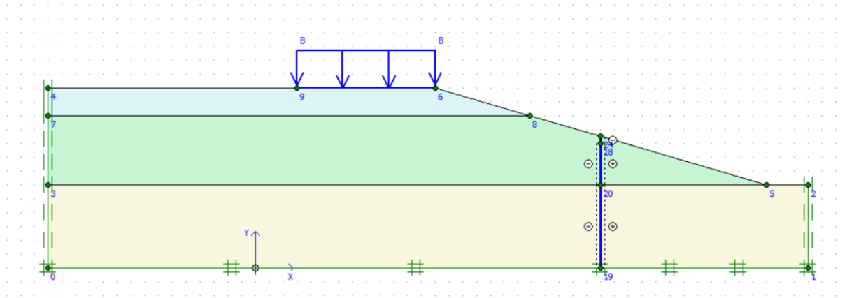
Gambar 8 Permodelan Lereng Input Plaxis (Sumber : Hasil Analisis, Plaxis 8.6 ,2023)
