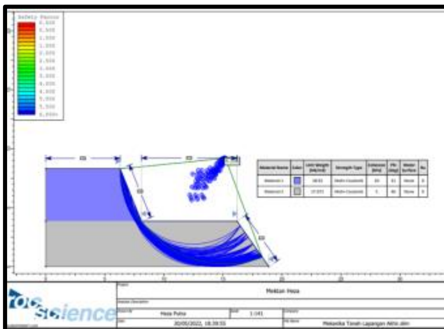
Gambar 6. Hasil analisis kestabilan seluruh lereng metode bishop
