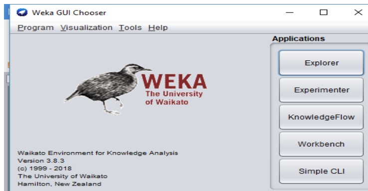
Gambar 2. Aplikasi Weka
