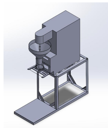
Gambar 6. Desain CAD alat cetak cilok.
