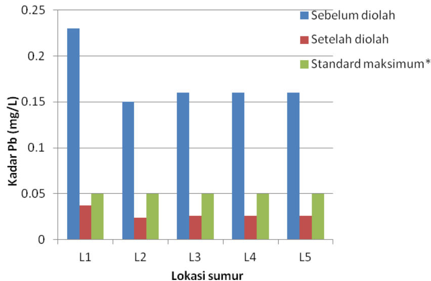
Gambar 6. Kandungan Pb pada 5 sampel air sumur sebelum dan setelah diolah menggunakan koagulan \text{FeCl}_3 1000 mg/L dibandingkan dengan standard maksimum
