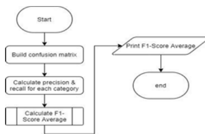
Gambar 6. Flowchart Evaluasi
