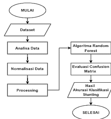
Gambar 3. Perancangan Sistem
