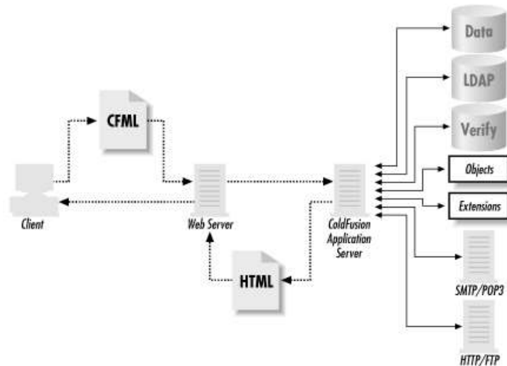
Gambar 1. Tahapan Permintaan ColdFusion Diproses
