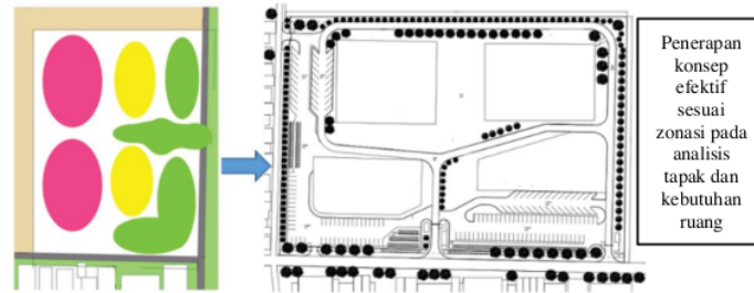
Gambar 4. Transformasi Lahan.
