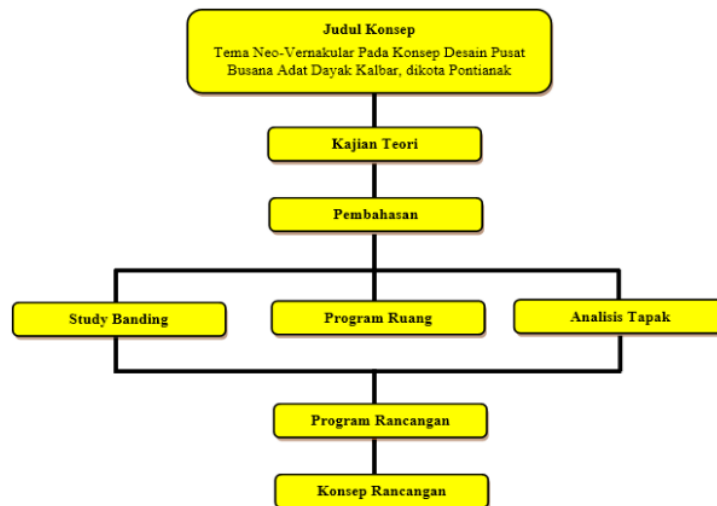
Gambar 1. Diagram Metodologi
