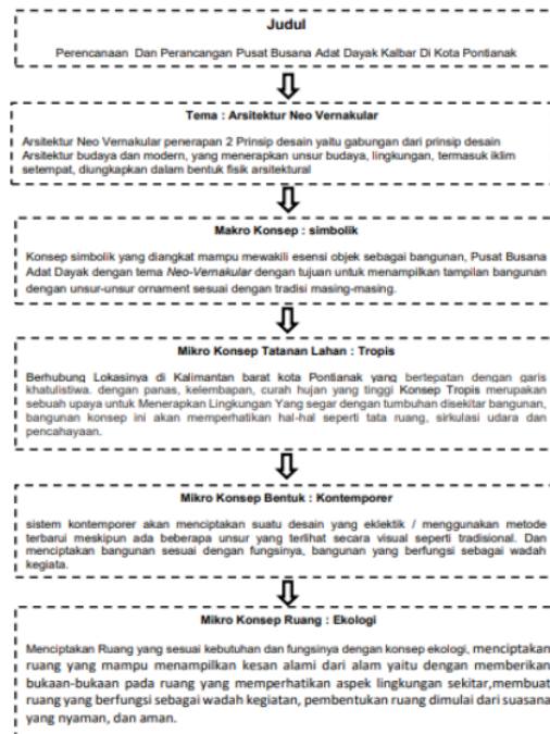
Gambar 8. Hirarki Konsep
