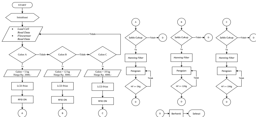
Gambar 4. Flowchart keseluruhan
