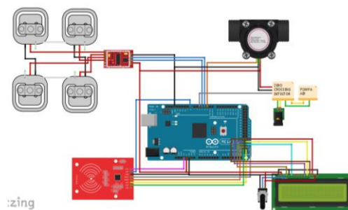
Gambar 3. Rangkaian Keseluruhan
