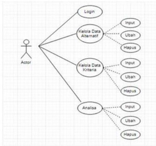
Gambar 3.2 Use Case Diagram Sistem Usulan Pemilihan Guru Terbaik
